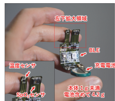
図2 シート型・血中酸素飽和度センサ
