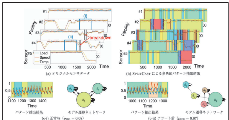
図3 工場設備センサデータに対するイベント予測技術
